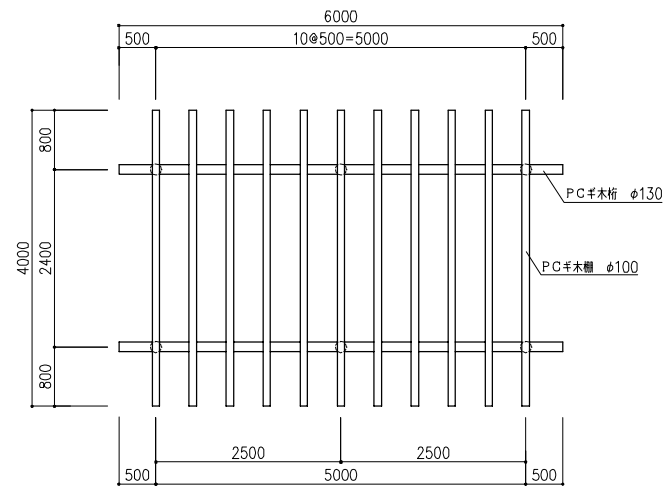
平面図 S=1:50
