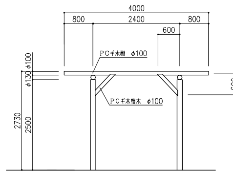
側面図 S=1:50
