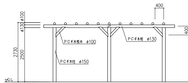
正面図 S=1:50
