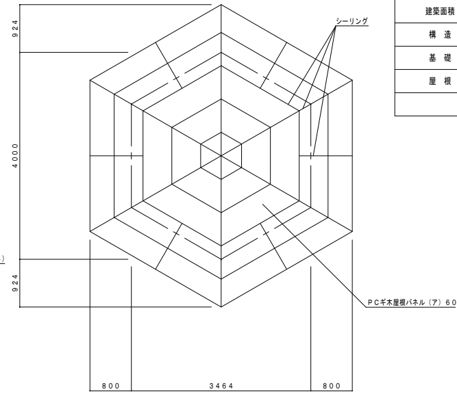
屋根伏図 S=1:50
