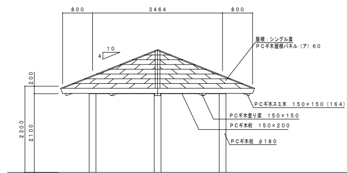
立面図 S=1:50
