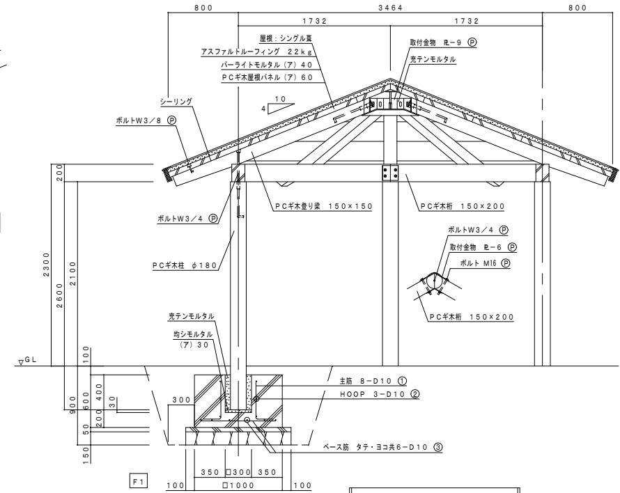
縦計図 S=1:30
