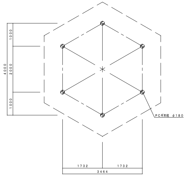
平面図 S=1:50
