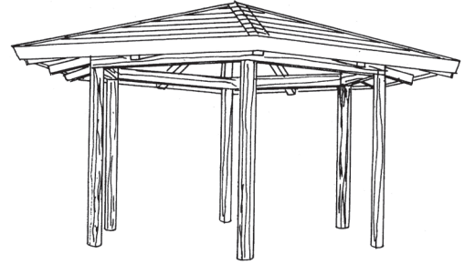
製品寸法/W:4,000 xL:3,464 xGLH:2,100 重量/6,810kg
