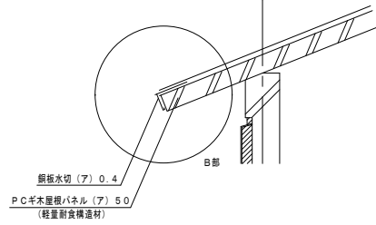
各部断面詳細図 S=1:10
