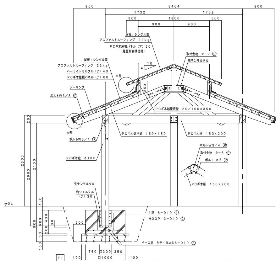
断面図 S=1:30
