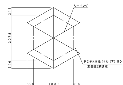
屋根桁伏図 S=1:50
