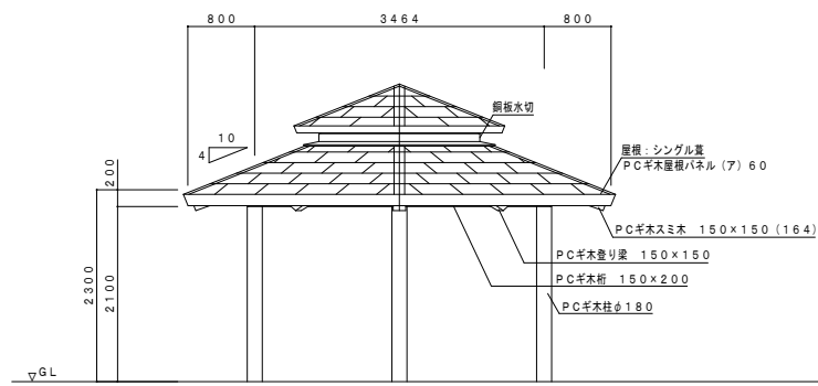
立面図 S=1:50
