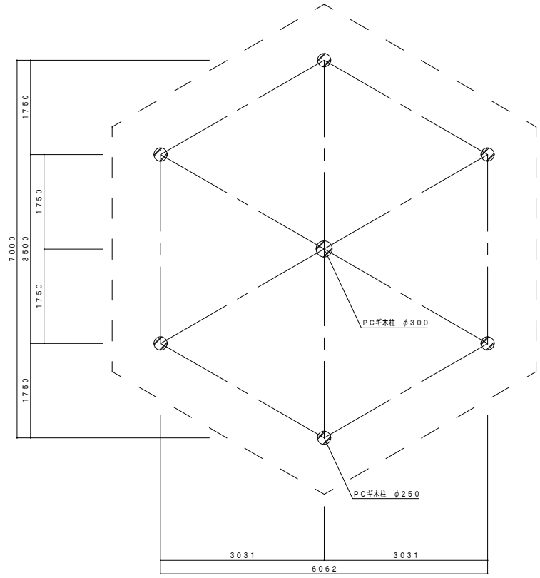
平面図 S=1:50
