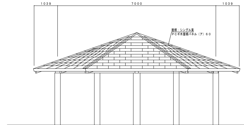
立面図 S=1:50
