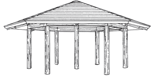
製品寸法/W:7,000 xL:6,062 xGLH:2,300 重量/17,161kg
