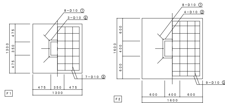
矩計図 S=1:30
