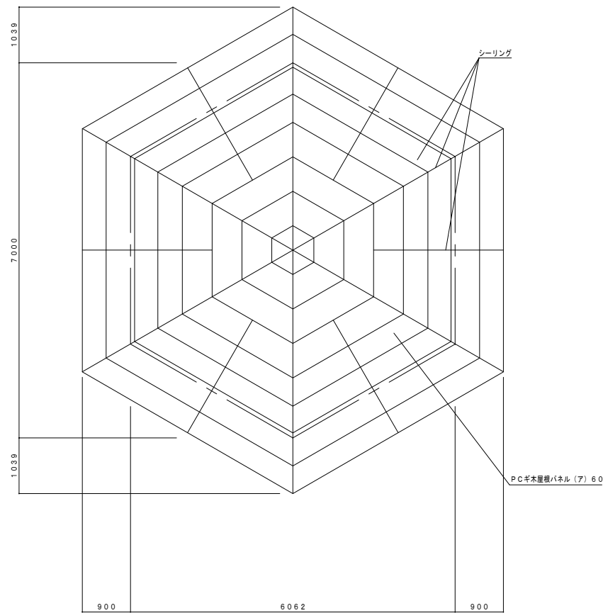
屋根伏図 S=1:50
