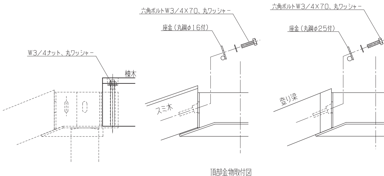
平面図 図-10
