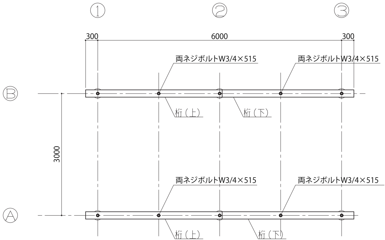
平面図
