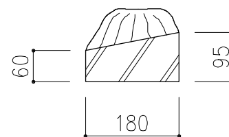
側面図
