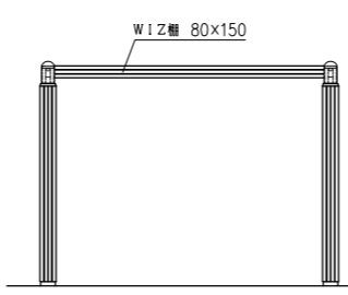
側面図 S=1:50
