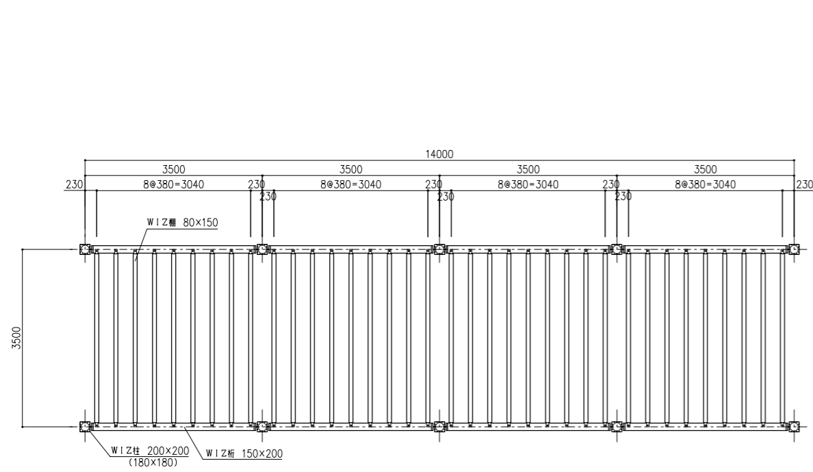
平面図 S=1:50
