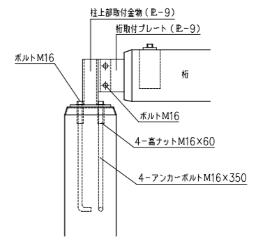
柱上部詳細図 S=1:10
