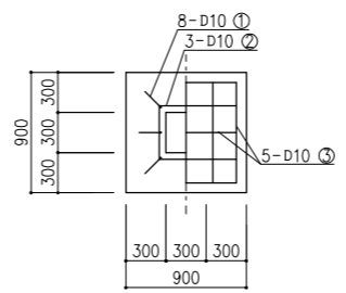
断面詳細図 S=1:30
