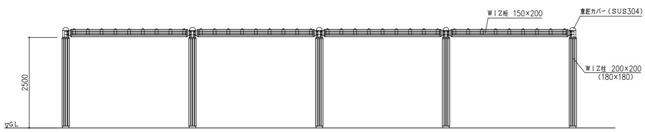
正面図 S=1:50
